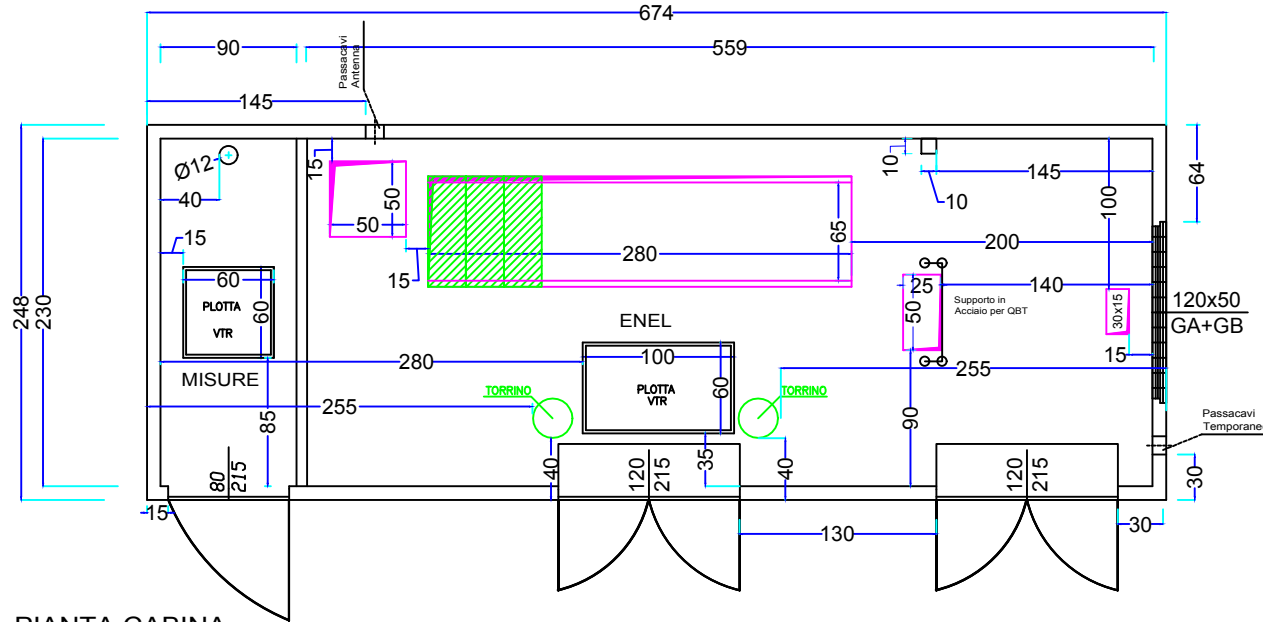
PIANTA CABINA
