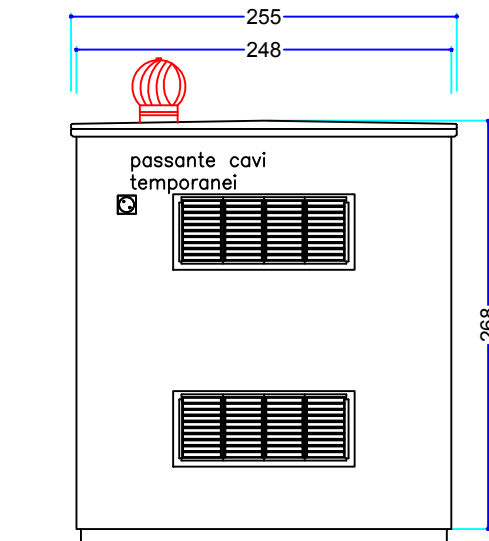
PROSPETTO DESTRO
