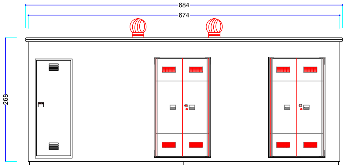
PROSPETTO FRONTALE
