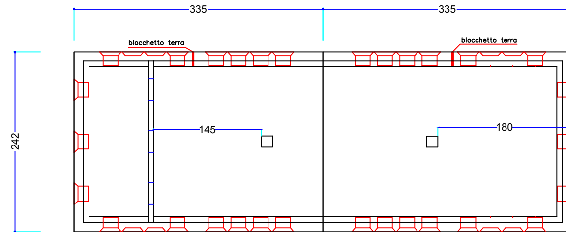
PIANTA BASE
