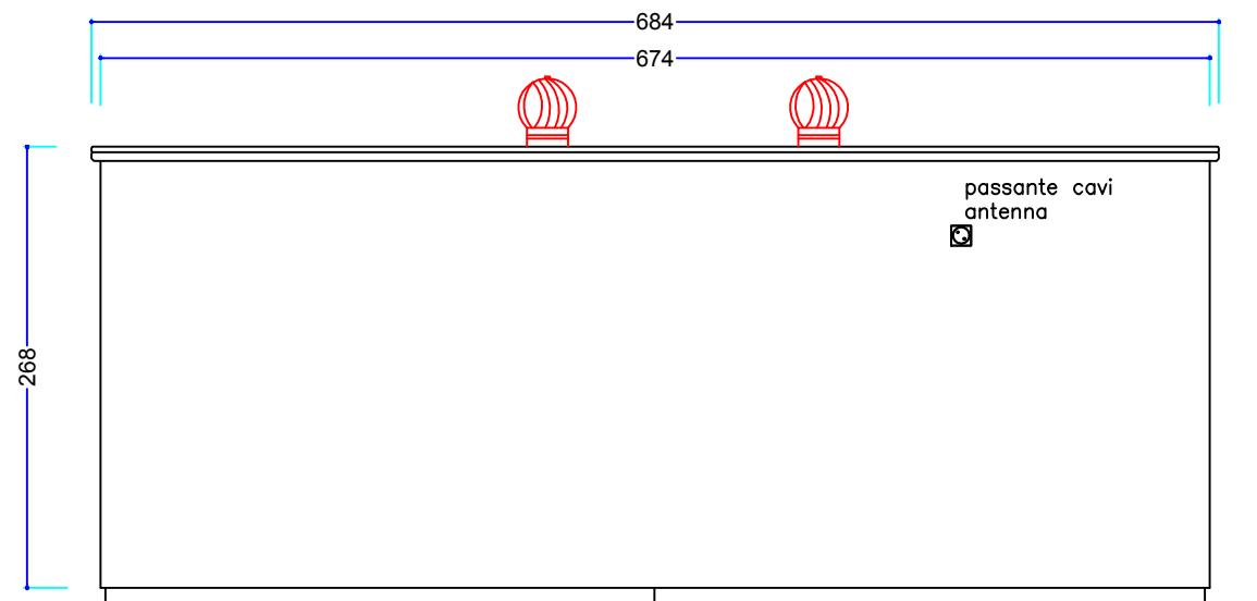
PROSPETTO TERGALE
